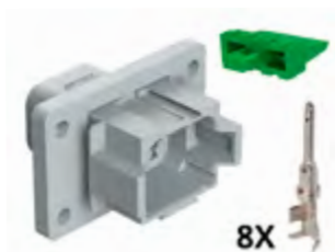
Conector AT04-08PA-L012 Macho - 8 Vias Cód. 1203083
