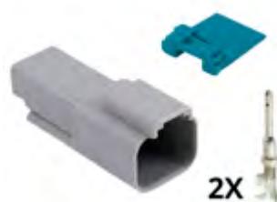
2X Conector DT04-2P Macho - 2 vias Cód. 1217021
