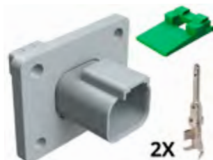
Conector AT04-2P-L012 Macho - 2 Vias Cód. 1203023
